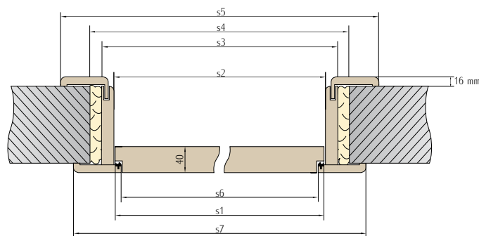
Schemat ościeżnicy regulowanej z odwrotną przylgą
