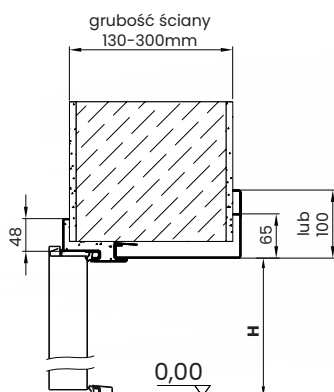
PRZEKRÓJ PIONOWY
