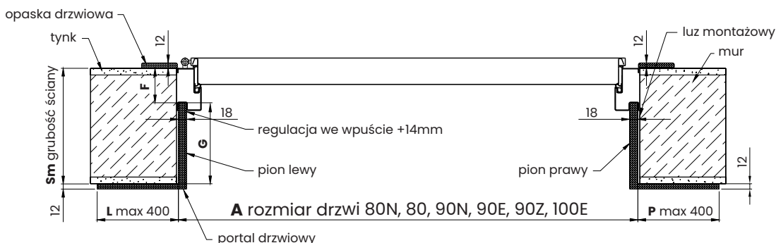
PRZEKRÓJ POZIOMY
