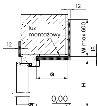
PRZEKRÓJ PIONOWY
