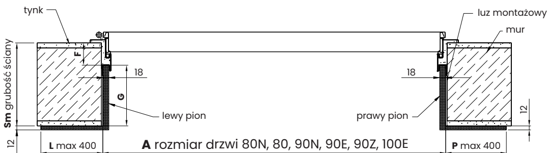
PRZEKRÓJ POZIOMY
