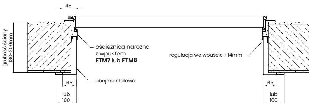
PRZEKRÓJ POZIOMY
