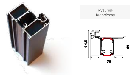
Ościeżnica aluminiowo-kompozytowa Premium
