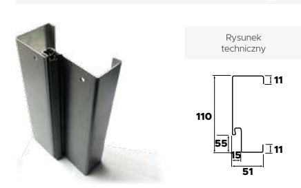
Ościeżnica "11" Protect
