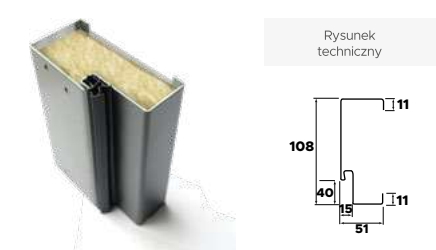
Ościeżnica kątowa Iron
