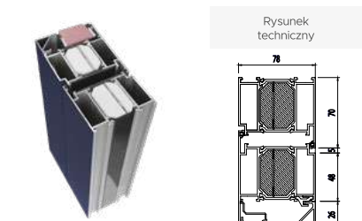
Ościeżnica Alu Hybrid
