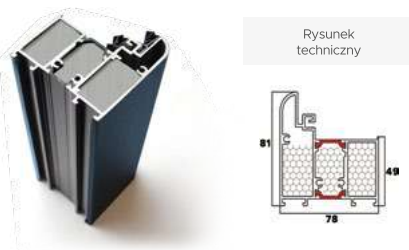
Ościeżnica aluminiowo-kompozytowa Optimum
