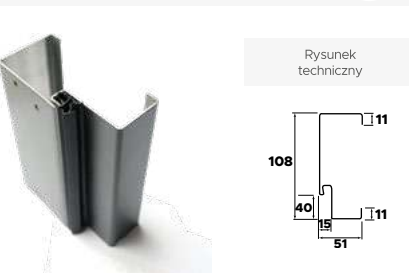
Przekrój drzwi ALU Fireline
