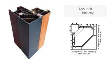
Ościeżnica symetryczna Iron
