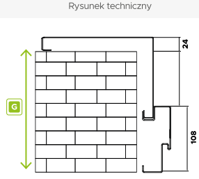
Portal z ościeżnicą wewnętrzną Iron
