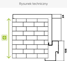
Portal z ościeżnicą regulowaną Iron
