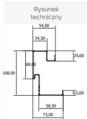
Ciepły próg PVC/ALU z przegrodą termiczną Prestige, Optimum, Premium Plus
