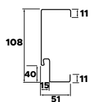
Rysunek techniczny
