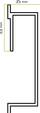
przekrój
