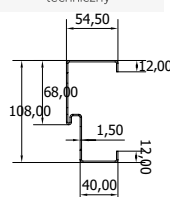
Rysunek techniczny
