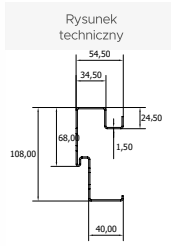
Próg aluminiowy Optimum,
