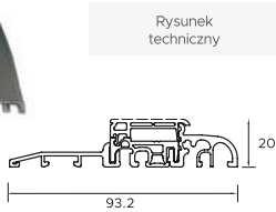
Ciepły próg PVC/ALU z przegrodą termiczną Alu Hybrid
