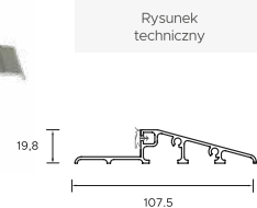
Próg aluminiowy z uszczelką Premium, Normal, Protect, Iron do ościeżnicy "9" (kątownej), "11" (wewnętrznej)
