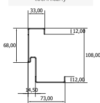
Rysunek techniczny
