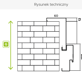
Opaska z ościeżnicą wewnętrzną Iron
