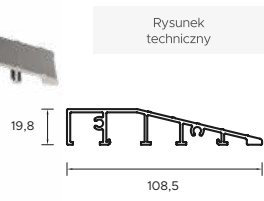
Próg aluminiowy Optimum,
