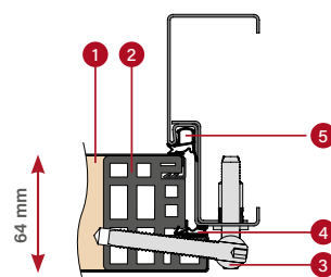
OŚCIEŻNICA STAŁOWA
